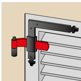
41PA5EJ. Rollenstück Aluminium, gerollt, gekröpft, 39x5 Ø14 Nœud aluminium roulé, coudé, 39x5 Ø14 Nodo estruso alluminio, ad angolo non forato 39x5 Ø14
