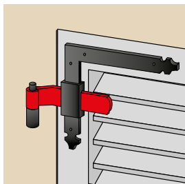
41PA76J. Rollenstück Aluminium, gerollt, gekröpft, 39x4 Ø14 Nœud aluminium roulé, coudé, 39x4 Ø14 Nodo estruso alluminio, ad angolo non forato 39x4 Ø14
