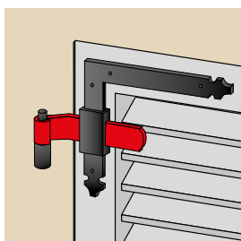
41PA5FJ. Rollenstück Aluminium, gerollt, gekröpft, 39x5 Ø16 Nœud aluminium roulé, coudé, 39x5 Ø16 Nodo alluminio sagomato non forato ad angolo 39x5 Ø16
