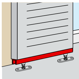
8501610 Führungsschiene, «U», Aluminium, 16 mm für Elastomerolive 850121C
